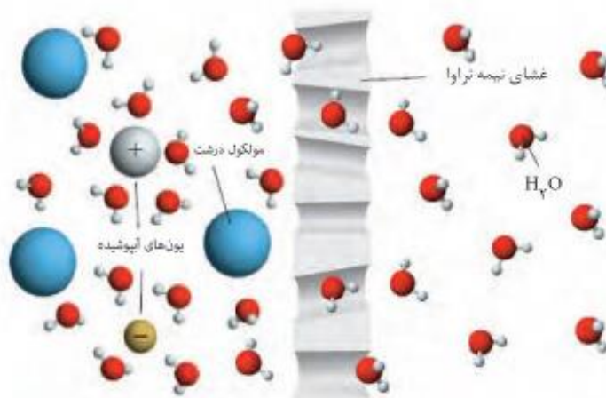
شکل ۲۹- غشای نیمه تراوا و عبور انتخابی
